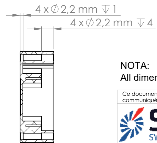
SECTION A-A SCALE 3 : 2.2
